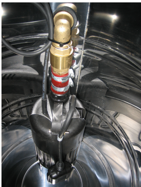
Potopna črpalka s plovcem
